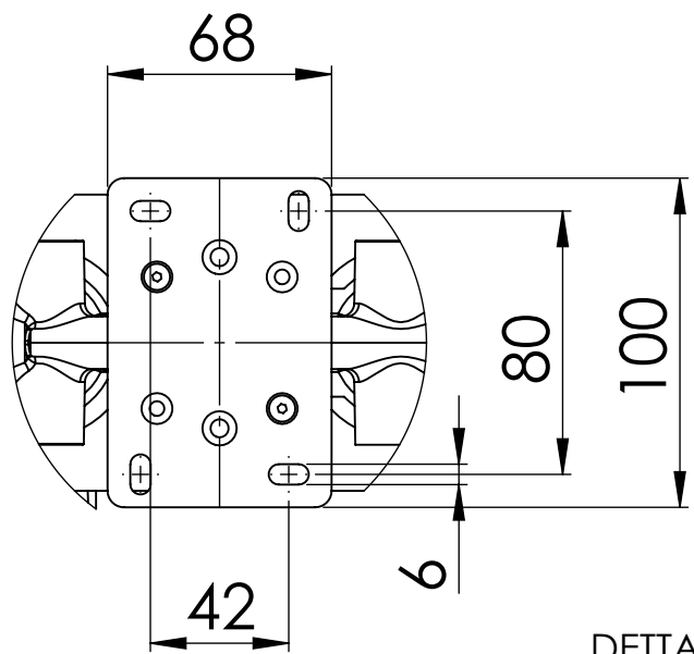
DETTAGLIO A SCALA 2 : 5
