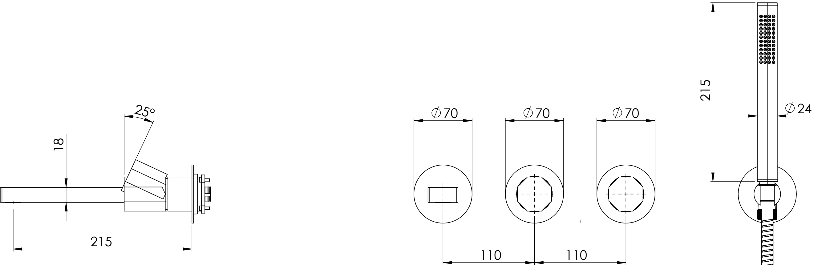
CONNESSIONE DEVIATORE D522AWBAB CONNECTION DIVERTER D522AWBAB
